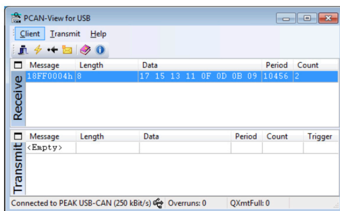
Figura 8.6 Ricezione di un Messaggio dei Codici di Risultato del Test
