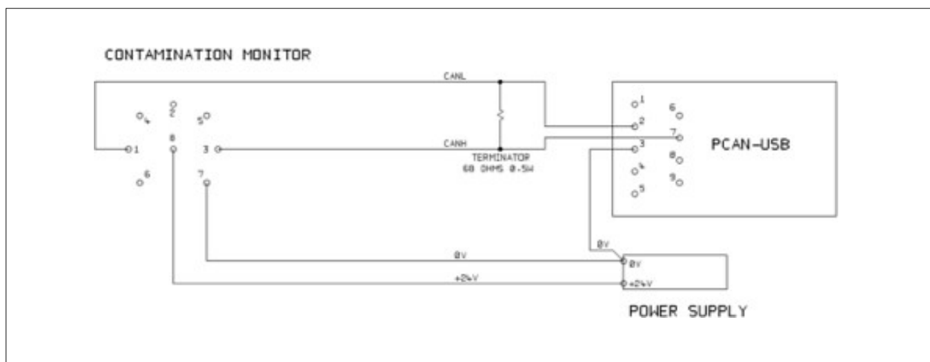
Figura 9.2 Collegamento dell'ICM 4.0 all'adattatore PCAN-USB
